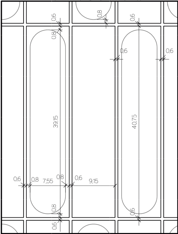
DETALLE FRONTAL Duelas forrado PANEL 1
